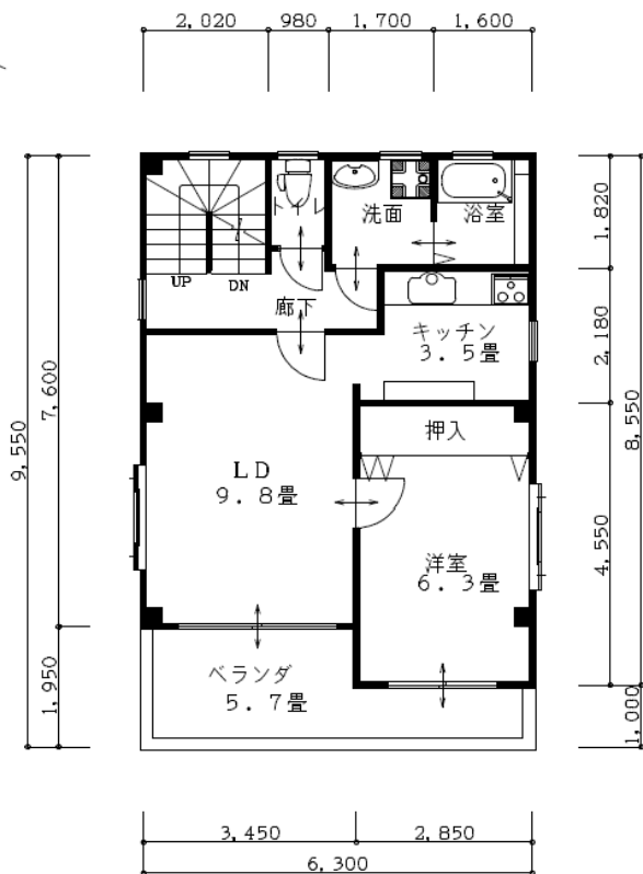
2 階平面図
