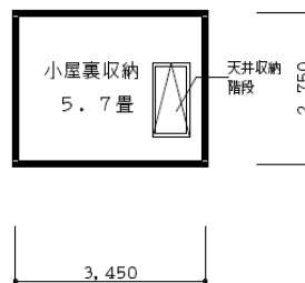
小屋裏平面図
