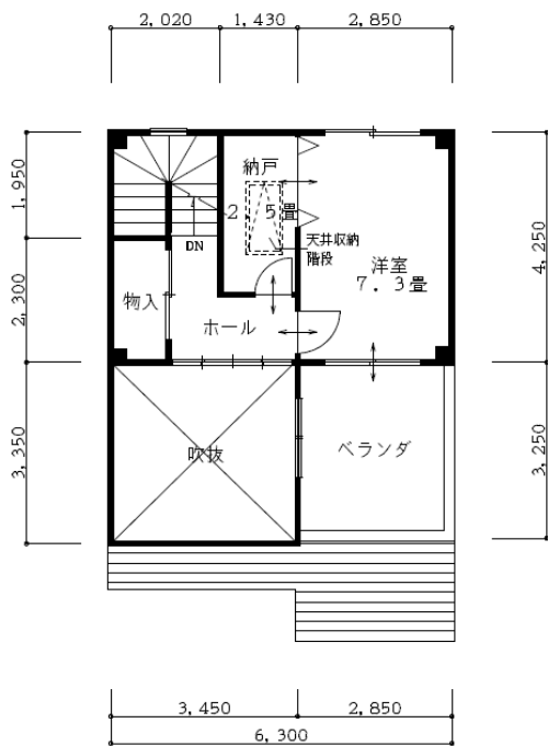
3 階平面図
